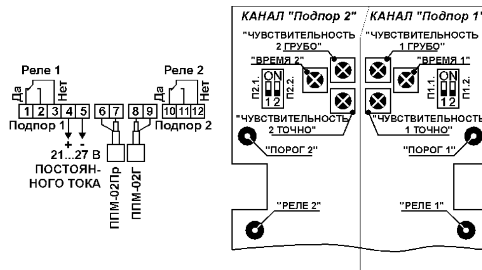
Рис. 7. Схема подключения и органы регулировки датчика РСУ-2А.
