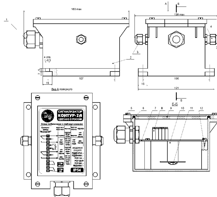
Рис. 1. Конструкция сигнализатора «Контур-2А» (модификация «РСУ-2А»).
