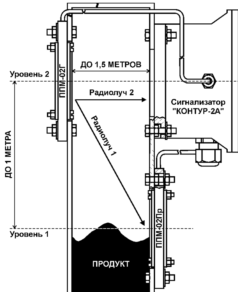
Рис. 3. Принцип действия сигнализатора РСУ-2А.
